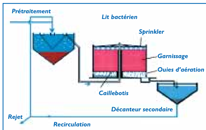
Figure n° 1 : Synoptique d'une station d'épuration comportant un lit bactérien (d'après site internet de Cartel : http://www.oieau.fr/ - rubrique guide des services - )
