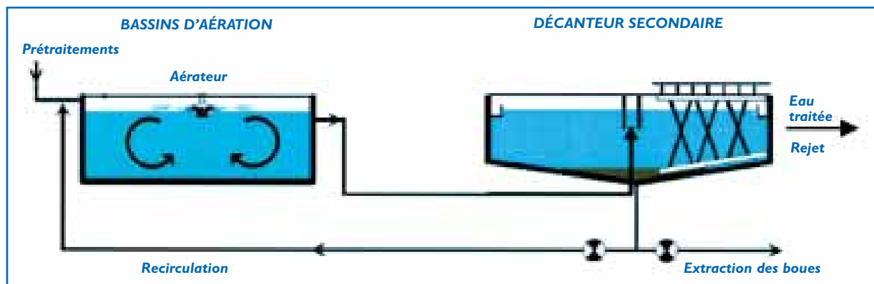
Figure n° 4 : Synoptique d'une boue activée - aération prolongée (d'après site internet de Cartel : http://www.oieau.fr/ - rubrique guide des services - )
