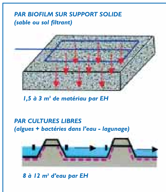
Figure n° 5 : Epuration "naturelle" extensive des eaux usées (Jean Duchemin, Commission Européenne - 2001)
