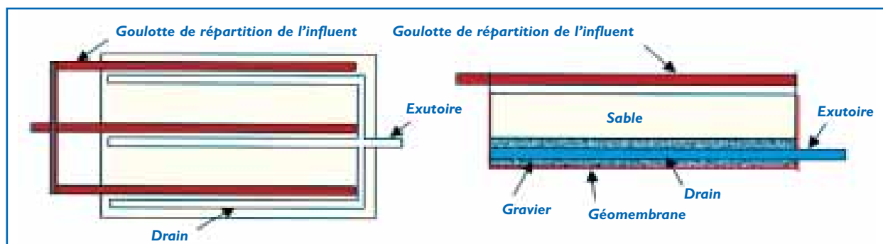
Figure n° 6 : Infiltration-percolation étanchée et drainée (Agences de l'Eau, 1993)
