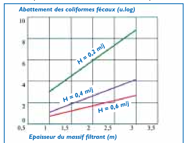
Figure n° 9 : Abattement des coliformes fécaux en fonction de la charge hydraulique (H en m/lj) et de l'épaisseur du massif filtrant
