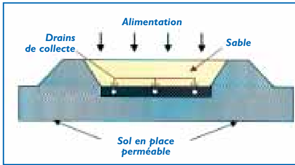
Figure n° 7 : Système drainé sur sol en place perméable (Agences de l'Eau, 1993)
