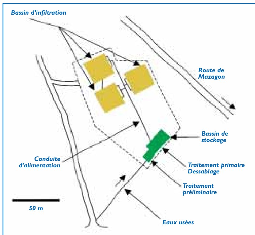
Figure n° 16 : Schéma de l'installation (V. Mottier, F. Brissaud, P. Nieto and Z. Alamy - 2000)
