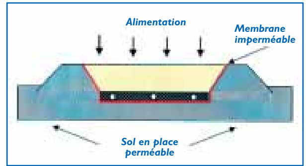
Figure n° 8 : Système drainé avec un massif drainant étanché par une membrane imperméable (Agences de l'Eau, 1993)
