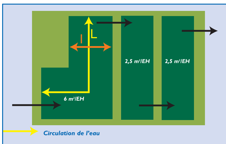
Figure n° 13 : Emprise au sol d'un lagunage naturel (Agence de l'Eau Seine-Normandie, CEMAGREF - 1998)
