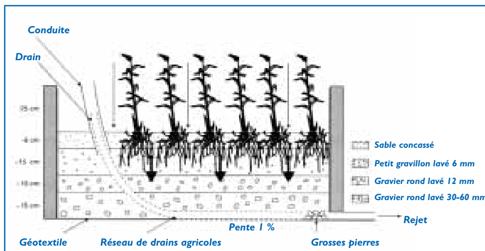
Figure n° 19 : Coupe des étages de filtres verticaux
