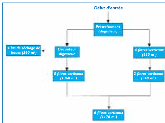
Figure n° 17 : Schéma de la filière (Montgomery Watson - 1997)
