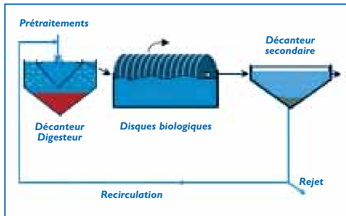
Figure n° 2 : Synoptique d'une station d'épuration comportant un disque biologique (d'après site internet de Cartel : http://www.oieau.fr/ - rubrique guide des services - )
