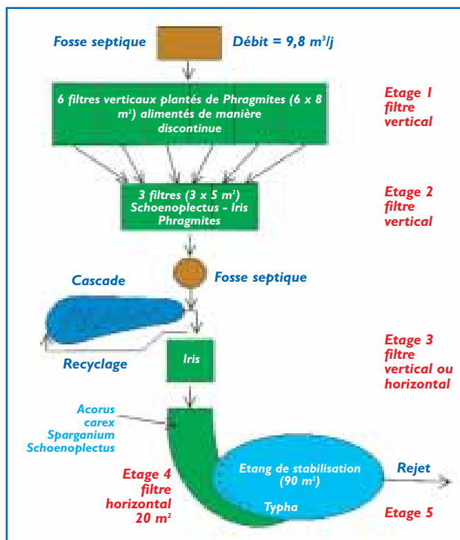
Figure n° 18 : Système mixte d'Oakland Park (Cooper et al, 1996)
